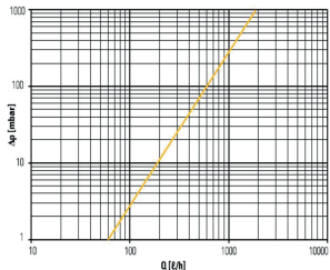
Gráfico: Pressão x Vazão da Desviadora
